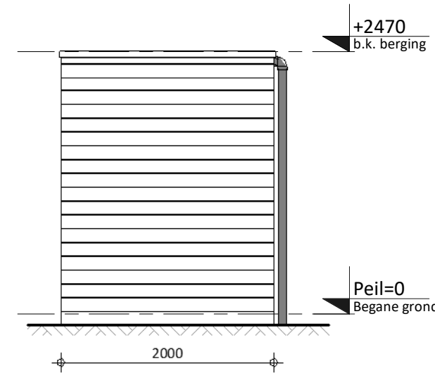
Linker zijaanzicht
