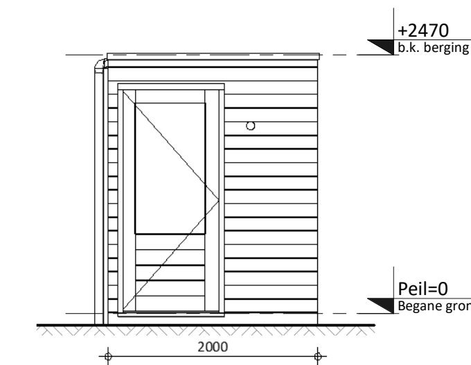
Rechter zijaanzicht
