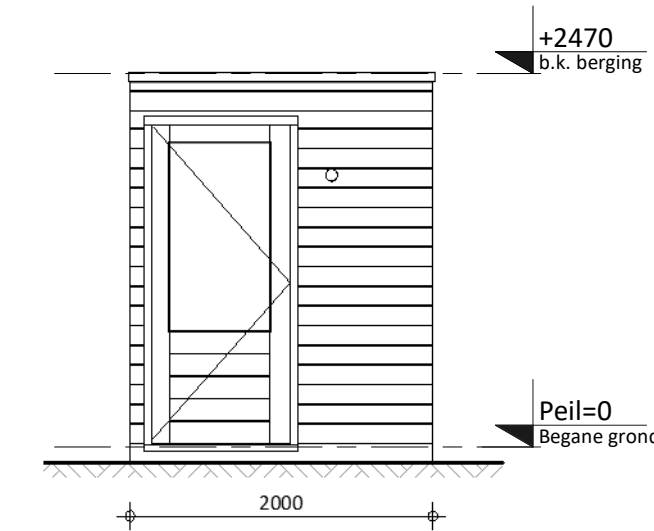
Rechter zijaanzicht
