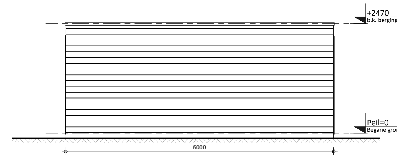
Achteraanzicht
