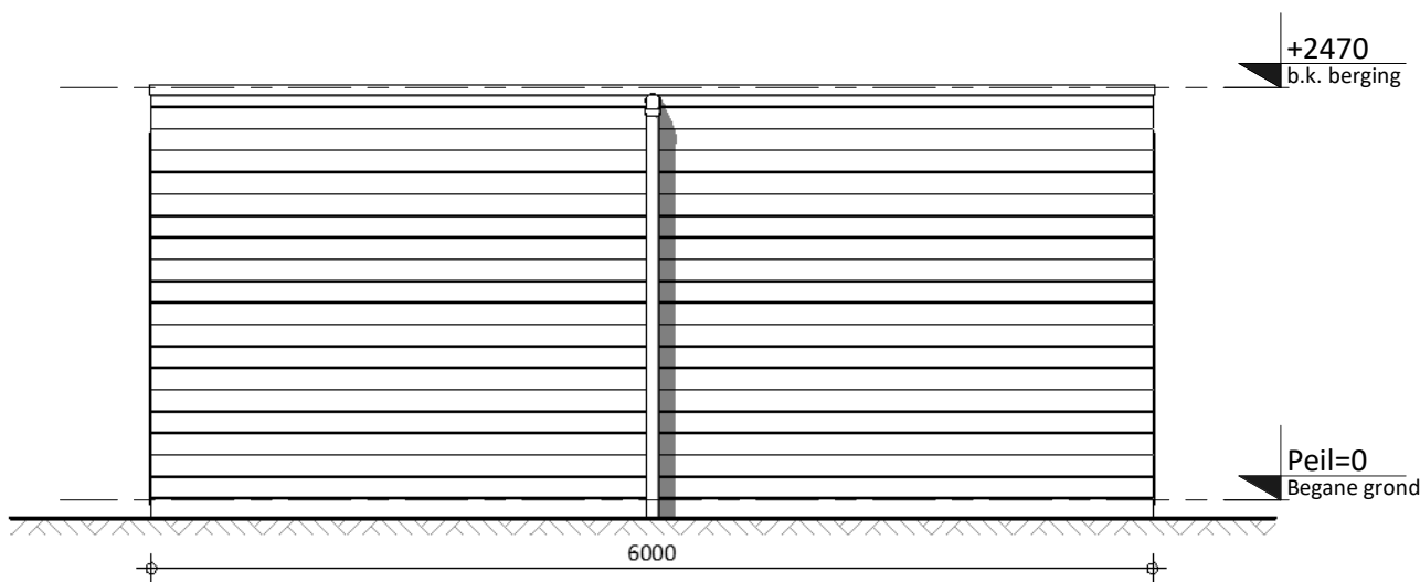
Vooraanzicht
