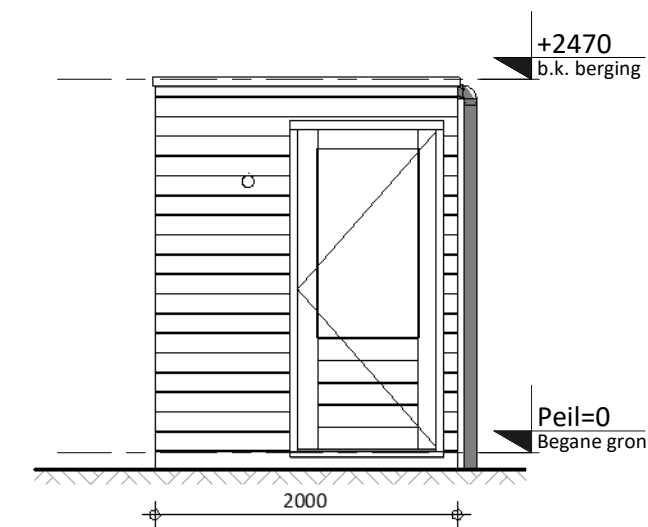
Linker zijaanzicht
