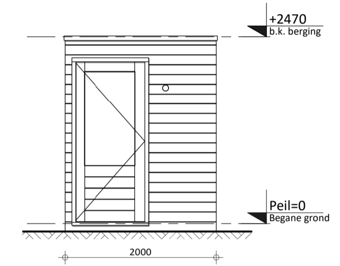
Rechter zijaanzicht
