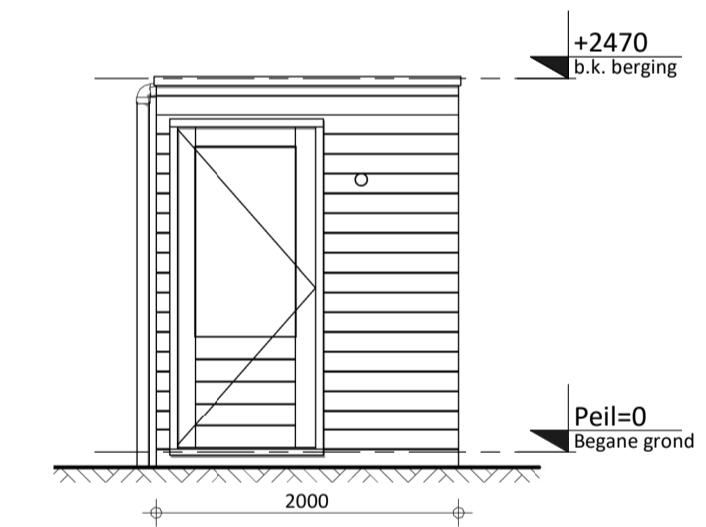
Rechter zijaanzicht
