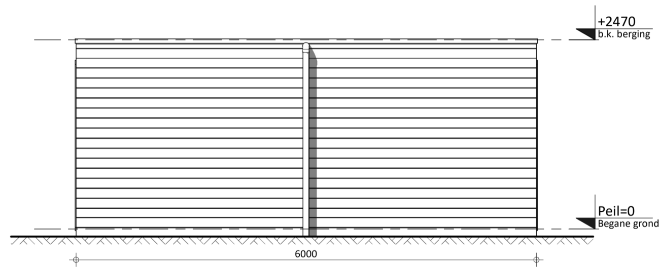
Vooraanzicht
